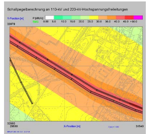
Schallpegelberechnung 1 m über dem Boden
