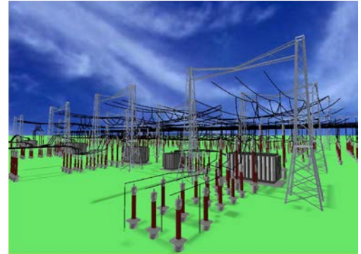
Magnetisches Feld an einer Schaltanlage
