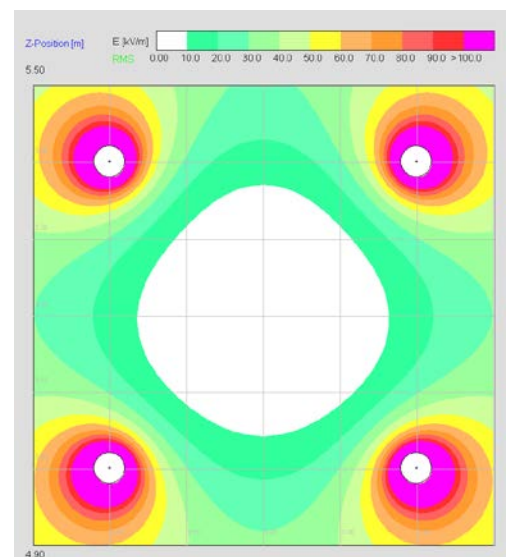
Randfeldstärken am Viererbündel
